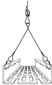
Y Accessoire embouts Maillon rapide sur chemins de câbles type fil
