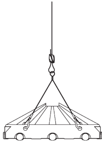
Y Accessoire embouts Crochets sur panneau radiant
